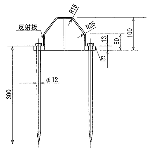
A-A' 断面図
