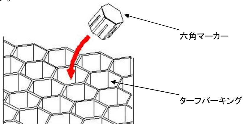
六角マーカース設置方法
